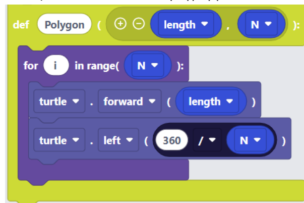
Εικόνα 2.8. Υποπρόγραμμα για το σχεδιασμό πολυγώνου
