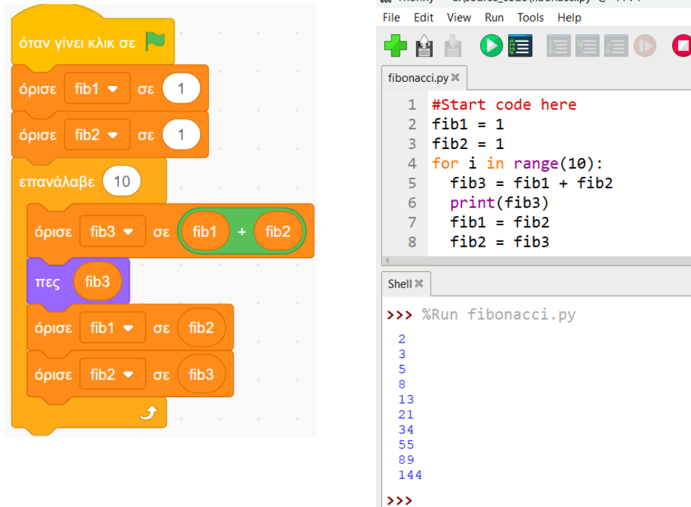
Εικόνα 2.5. Αλγόριθμος υπολογισμού των αριθμών Fibonacci στο περιβάλλον προγραμματισμού Scratch και στο περιβάλλον προγραμματισμού Thonny.
