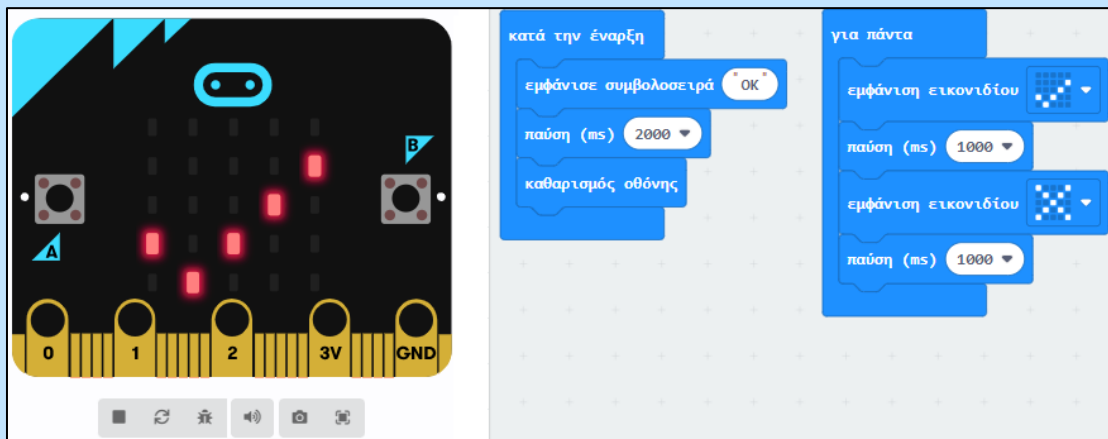
Εικόνα 3.7. Στιγμιότυπο του προγράμματος που εμφανίζει συμβολοσειρά και εικονίδια
