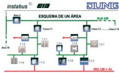
Εικόνα 45: Διάγραμμα διασύνδεσης συσκευών instabus
